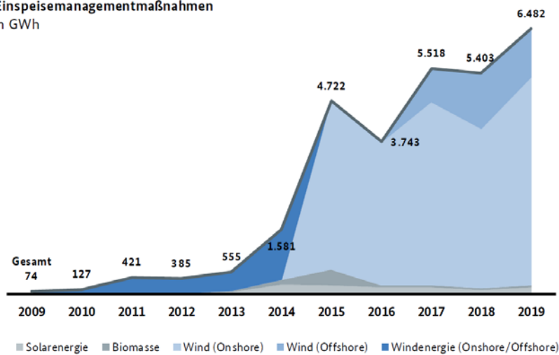
Abbildung 23: Abgeregelter elektrische Energie [BNA]
