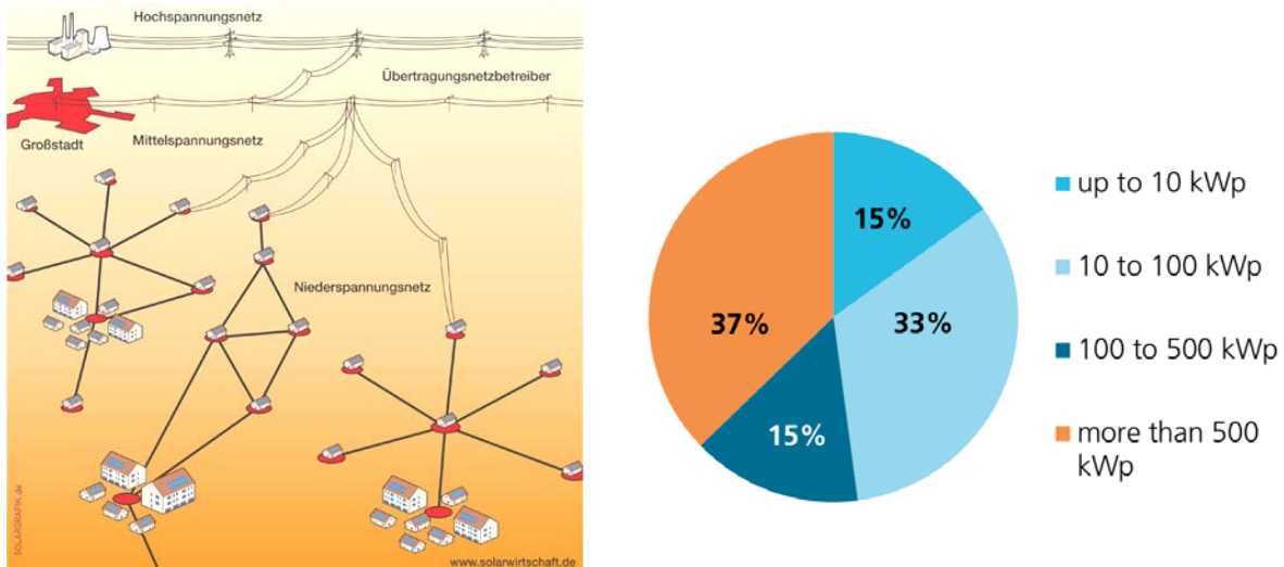
Abbildung 22: Links: Einspeisung von PV-Strom [BSW], Rechts: Verteilung der installierten PV-Leistung im Jahr 2020 nach Anlagengröße [ISE10]
