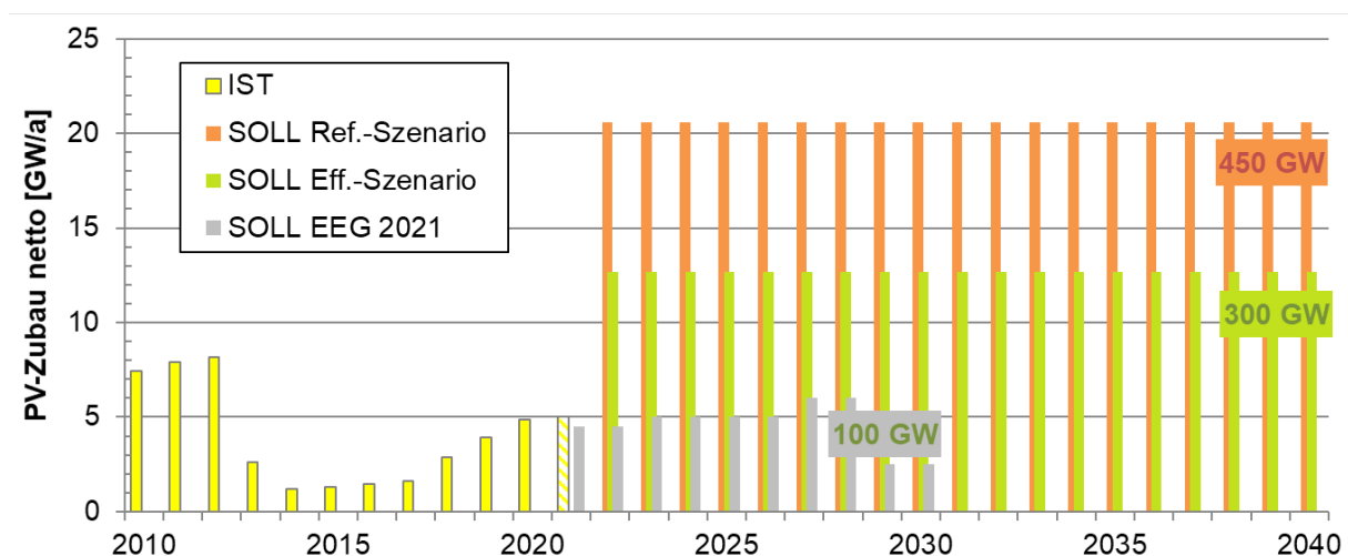
Abbildung 1: Netto-PV-Zubau: Istwerte bis 2020, Prognose für 2021, Zielwerte für gleichmäßigen Ausbau auf 300 bzw. 450 GW p und Zielwerte laut EEG 2021 (ohne Vorzieheffekte durch Sonderausschreibungen)
