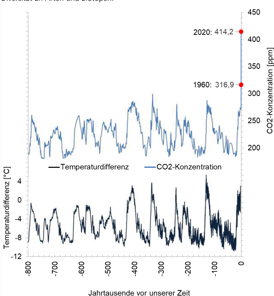
Abbildung 39: Schätzungen der atmosphärischen CO 2 -Konzentration und der Temperaturdifferenz in der Antarktis auf Basis von Eisbohrkernen [EPA]; Rot: zwei neuere CO 2 -Messwerte des Mauna Loa Observatory [ https://www.esrl.noaa.gov/gmd/ccgg/trends/data.html ]
