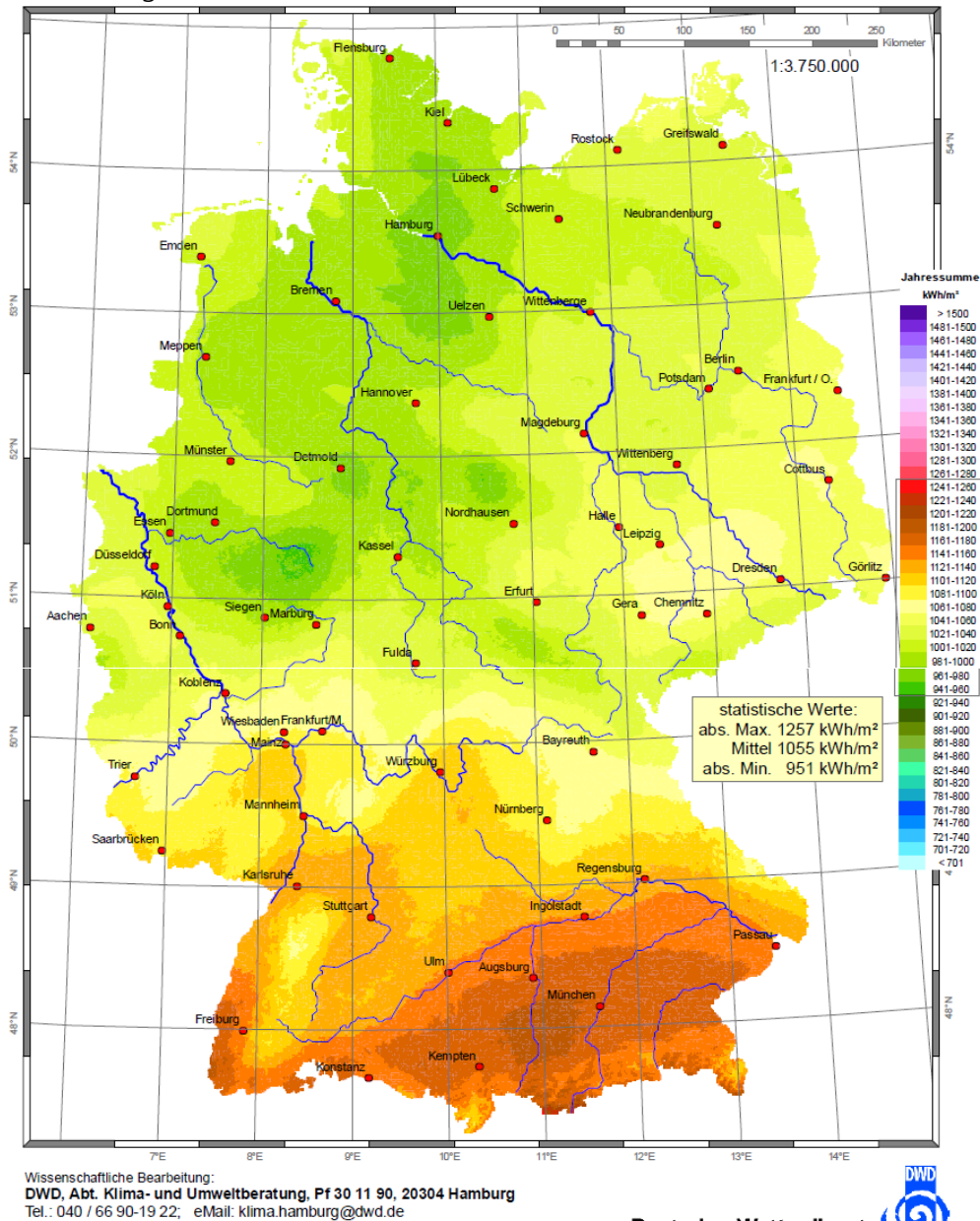
Abbildung 37: Horizontale jährliche Globalstrahlungssumme in Deutschland, gemittelt über den Zeitraum 1981-2010 [DWD]
