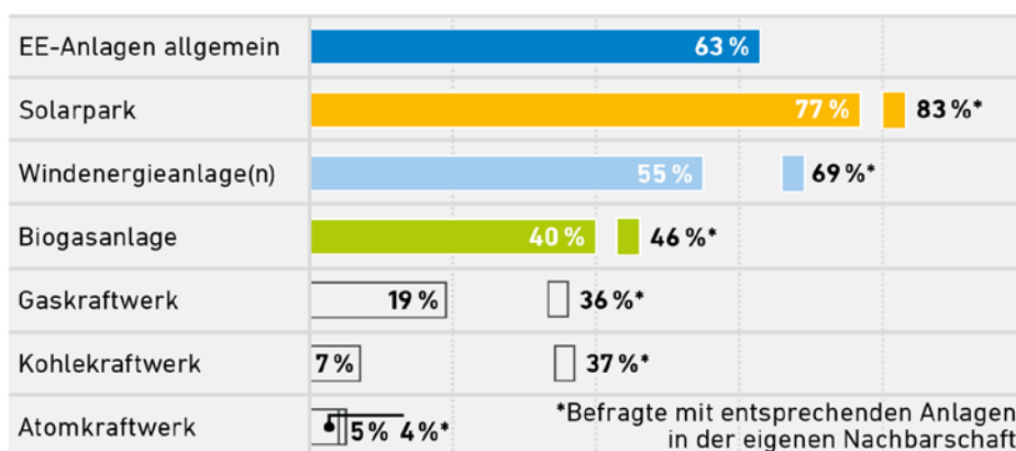
Abbildung 33: Umfrageergebnisse zur Akzeptanz verschiedener Kraftwerkstypen [AEE4]
