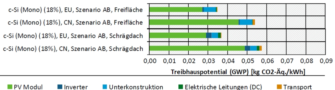
Abbildung 40: Treibhauspotential der Stromerzeugung mit mono c-Si PV für Dach- und Freiflächenanlagen [UBA7]
