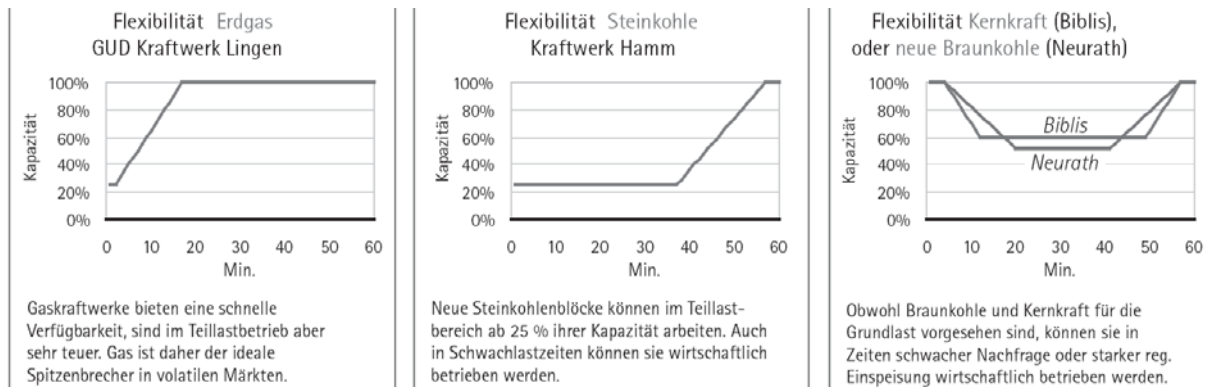
Abbildung 55: Verfügbarkeit von Kraftwerken [VGB]
