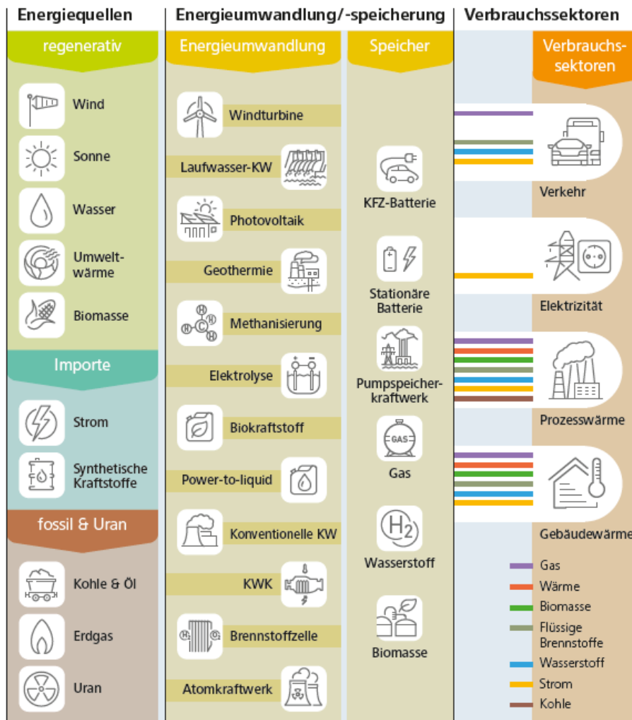
Abbildung 49: Schematische Darstellung des Modells REMod (KW: Kraftwerk, KWK: Kraft-Wärme-Kopplung, [ISE12])
